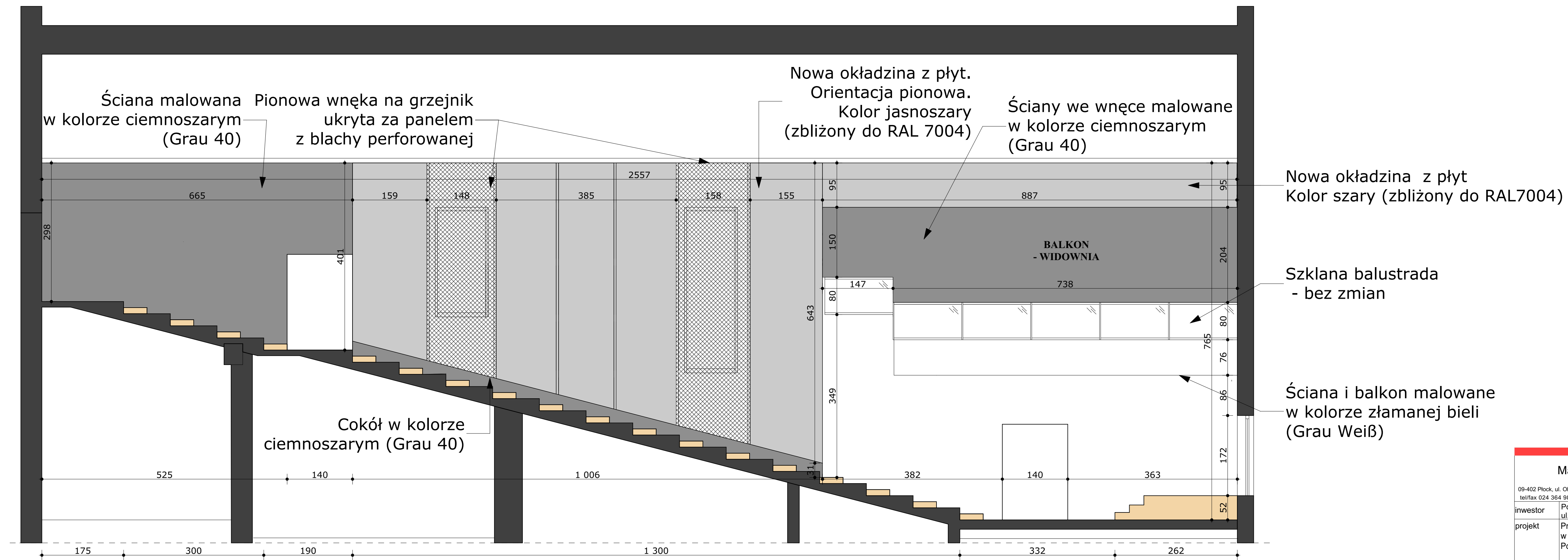
PRZEKRÓJ C-C
